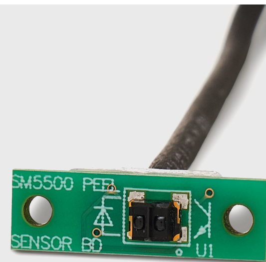
ОПТИЧЕСКИЙ ДАТЧИК С ПРОВОДОМ MOLEX, JST, 1.25MM
